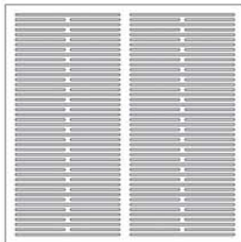
CLASSIC型 鏤空圖案吸音板 產品編碼： ASP-CL N.R.C. 0.90 (50mm) 吸音系數 0.95 (90mm*)
